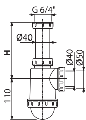
A443: H=70-180
